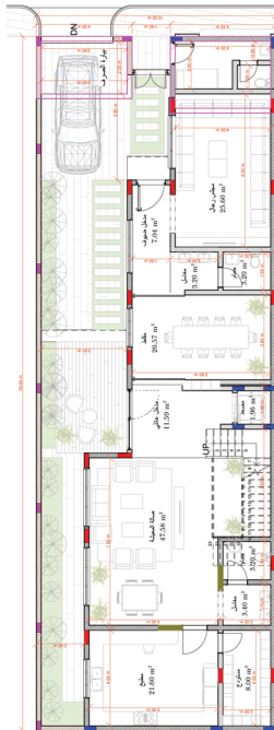
مخطط الدور الارضي
