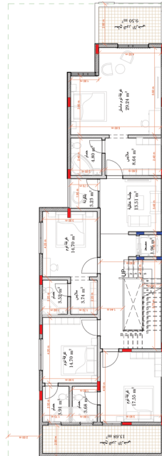
مخطط الدور الاول
